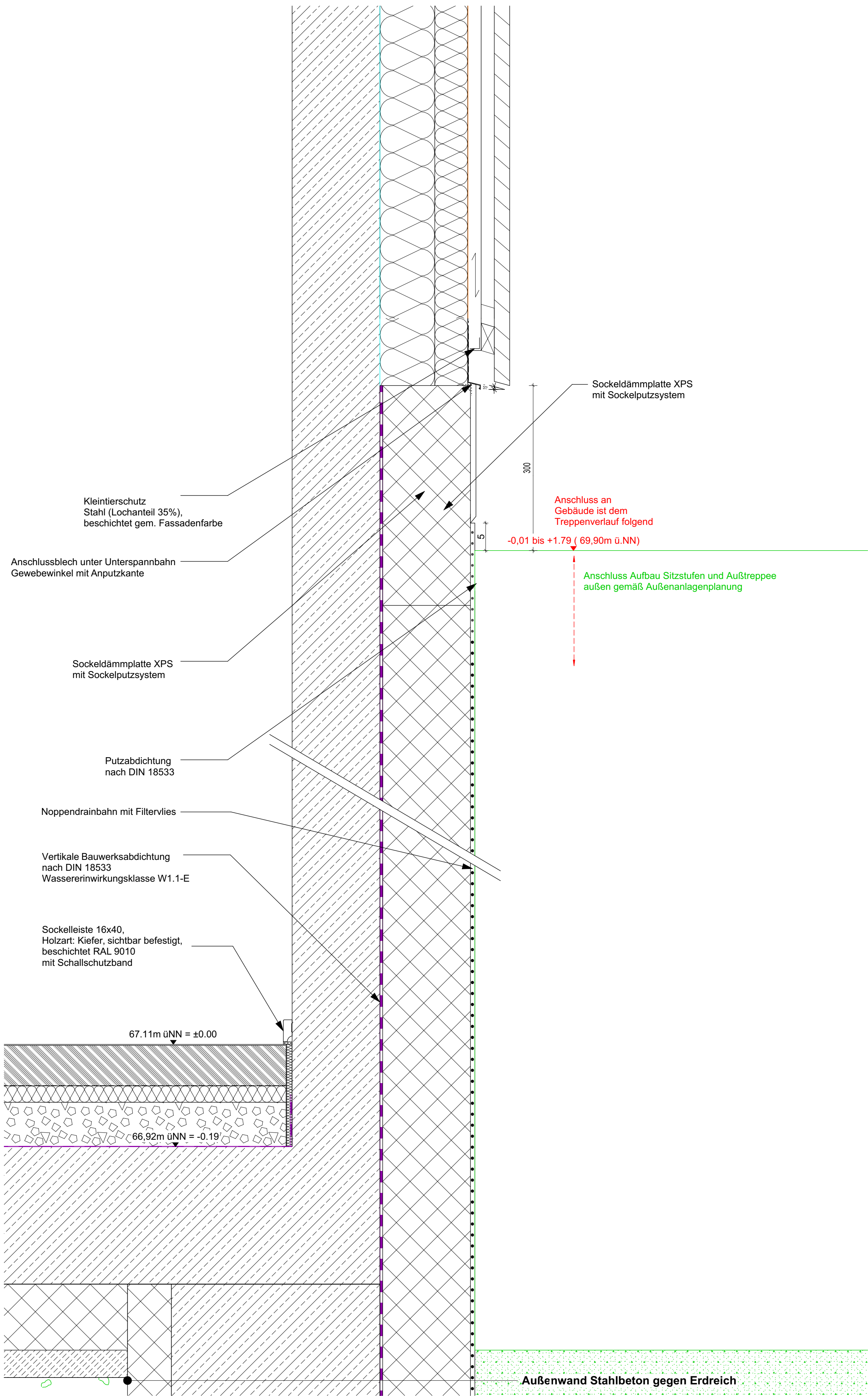
Sockeldetail Nordfassade - Außentreppenbereich
