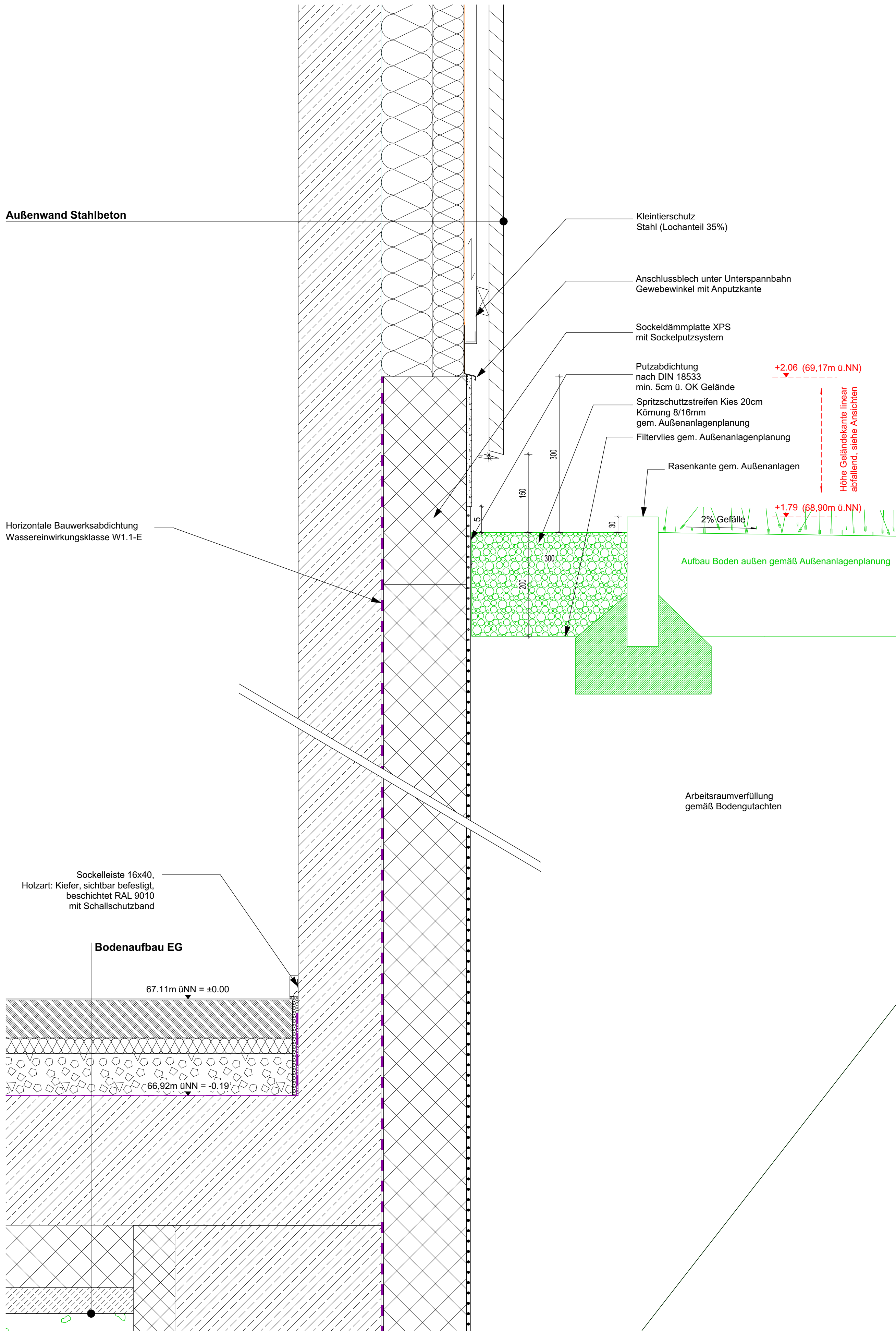
Sockeldetail Ostfassade - Kiesbett
